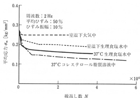
図 1・62 セグメント化ポリウレタン(東洋紡績 TM5)の疲労特性に及ぼす各種雰囲気の影響 39)
